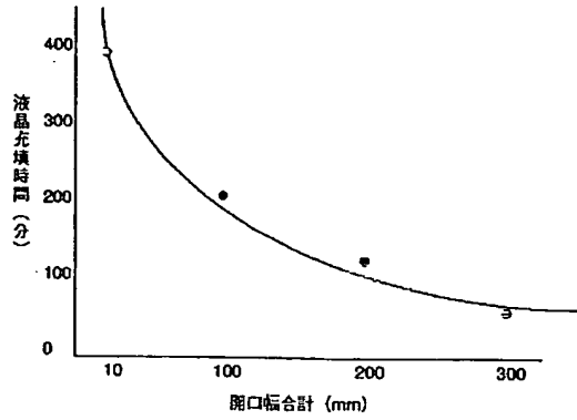
注入口の開口幅の合計と液晶充填時間との関係
